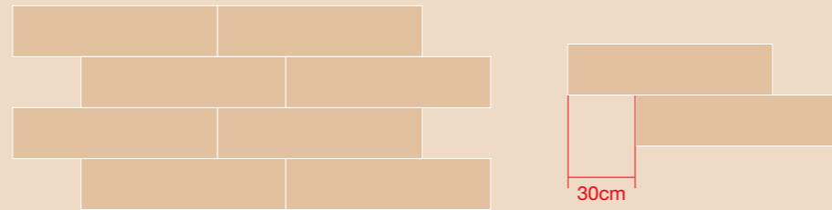
2-Укладка вразбежку с фиксированным смещением по два прямых ряда 2-Posa a modulo regolare a due file 2-Double file regular module installation pattern
