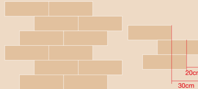
4-Укладка вразбежку с фиксированным смещением по три прямых ряда 4-Posa a modulo regolare a tre file 4-Triple file regular module installation pattern
