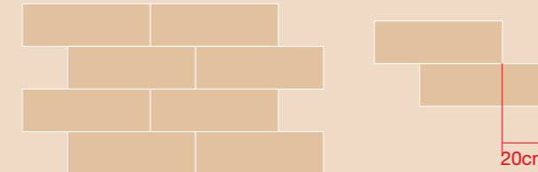
2-Укладка вразбежку с фиксированным смещением по два прямых ряда 2-Posa a modulo regolare a due file 2-Double file regular module installation pattern
