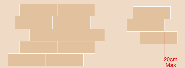
5-Укладка вразбежку с хаотичным смещением 5-Posa a modulo irregolare 5-Irregular module installation pattern
